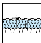
Flachdach ohne Schutz-, Beschwerungs- und Nutzschiicht (Nacktdach)
