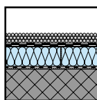
Flachdach im Verbund (Verbunddach)
