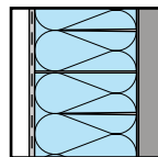
Aussendämmung verputzt
