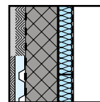
Innendämmung verputzt
