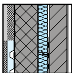
Kerndämmung
