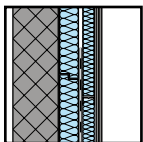
Innendämmung beplankt mit GKP auf C-Profil o.ä.
