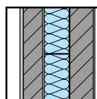
Kerndämmung
