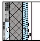
Innendämmung beplankt mit GKP o.ä.
