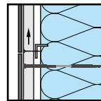
Fassadenbekleidung hinterlüftet / Unterkonstruktion
