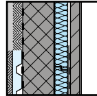
Innendämmung mit Vormauerung verputzt
