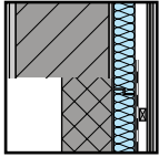
Innendämmung beplankt mit GKP auf Lattung o.ä.
