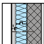
Aussendämmung hinterlüftet
