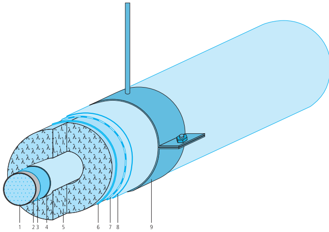
Bild 1.1-1: Prinzipieller Systemaufbau
